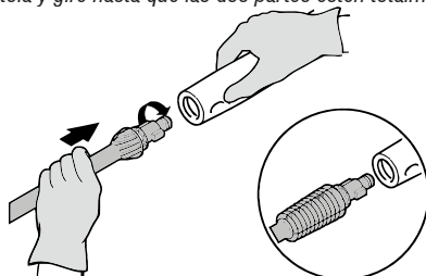
Figura 3 – Conectando la extensión en la lanza
