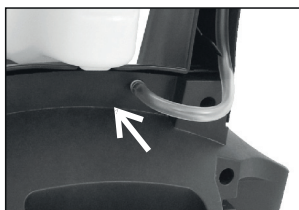
Figura 10 – Conexión de la manguera en el tanque de detergente
