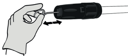
Figura 16 – Limpeza do bico da lança
