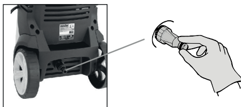
Figura 15 – Limpeza entrada de água
